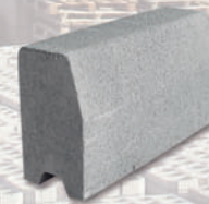
Bordillo 12x15x25x50 con ranura
