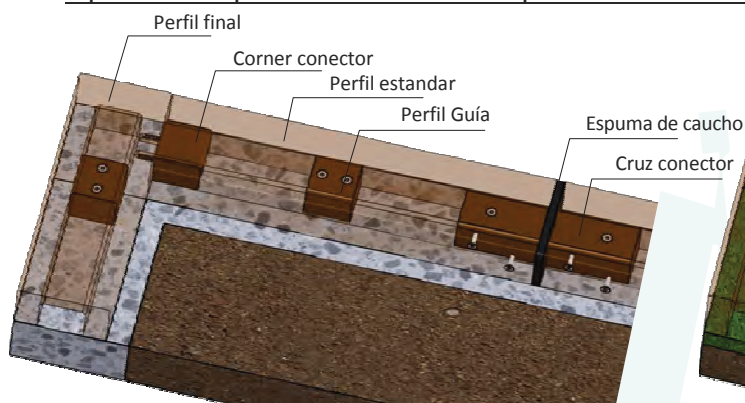
Representación esquemática de la instalación en superficie Secured
