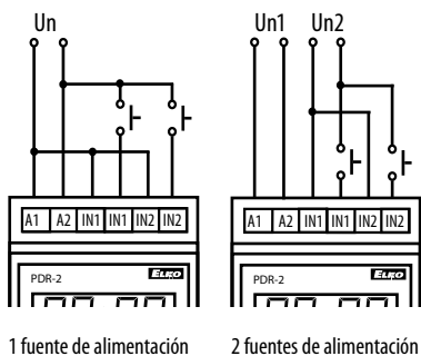
1 fuente de alimentación
