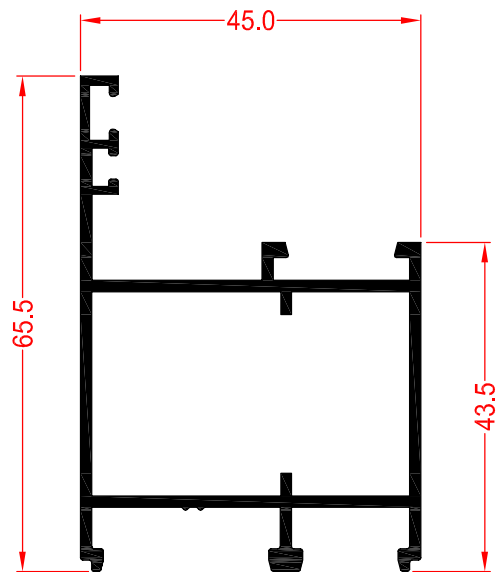
62702 CERCO PUERTA APERTURA EXTERIOR
