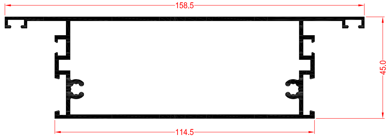
60538 TRAVESAÑO DE CERCO (158.5)
