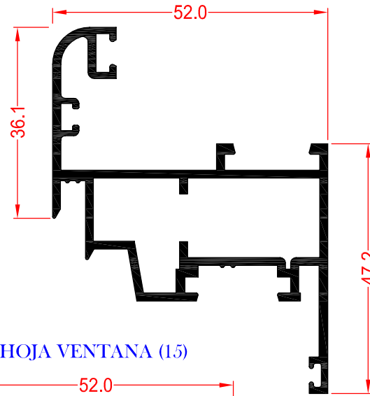
62673 HOJA CURVA VENTANA (15)
