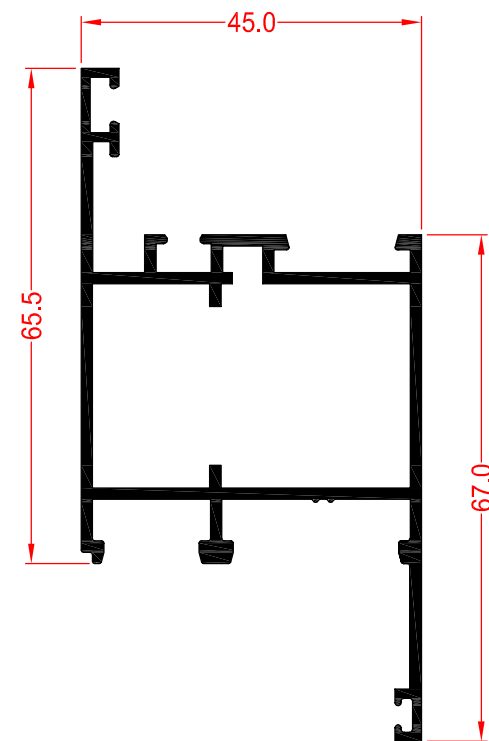
58960 CERCO PUERTA CON SOLAPE
