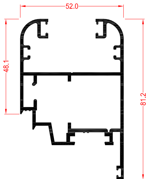
66605 HOJA CURVA SIN JUNQUILLO (27)
