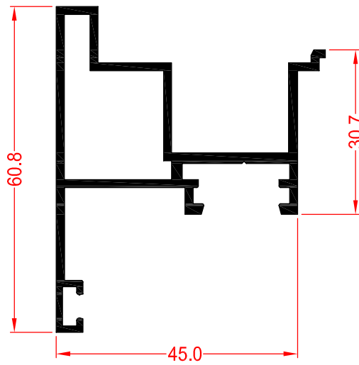
61140 INVERSOR APERT. EXTERIOR
