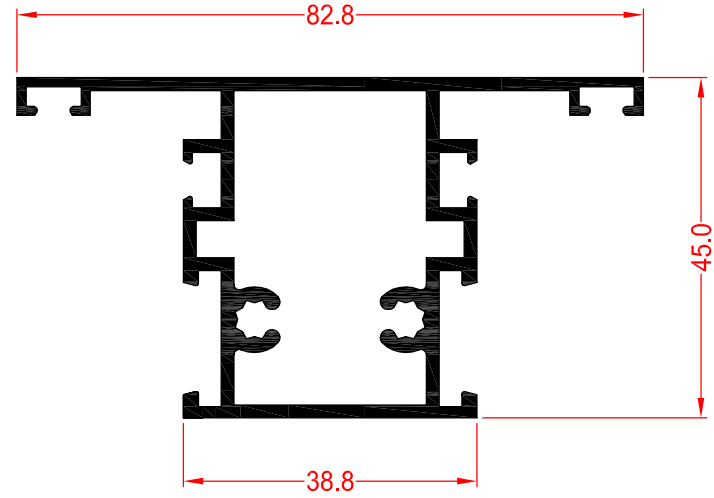
58961 TRAVESAÑO DE CERCO (83)
