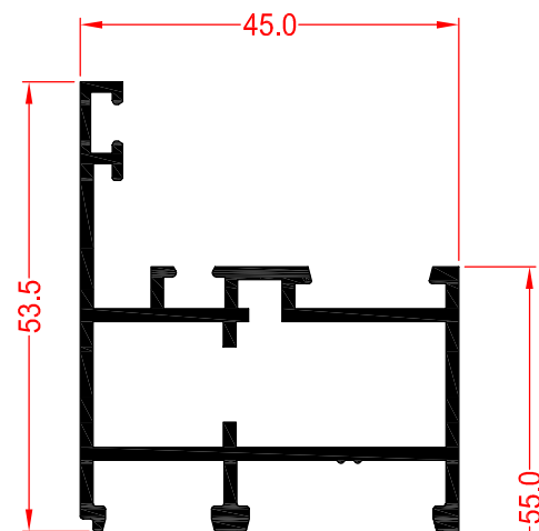
58956 CERCO VENTANA CON SOLAPE
