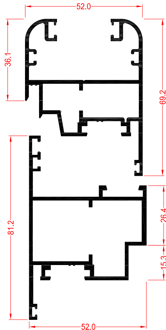
62092 HOJA APERTURA EXT. (27)
