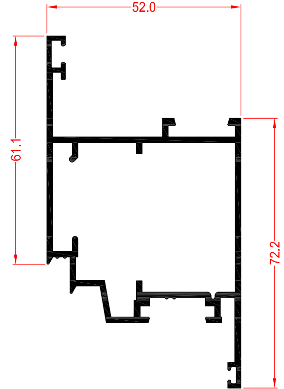
58963 HOJA PUERTA (40)
