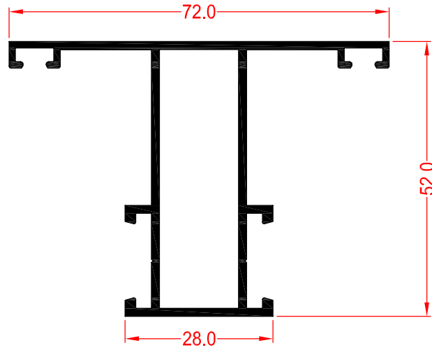
58953 TRAVESAÑO DE HOJA (158.5)
