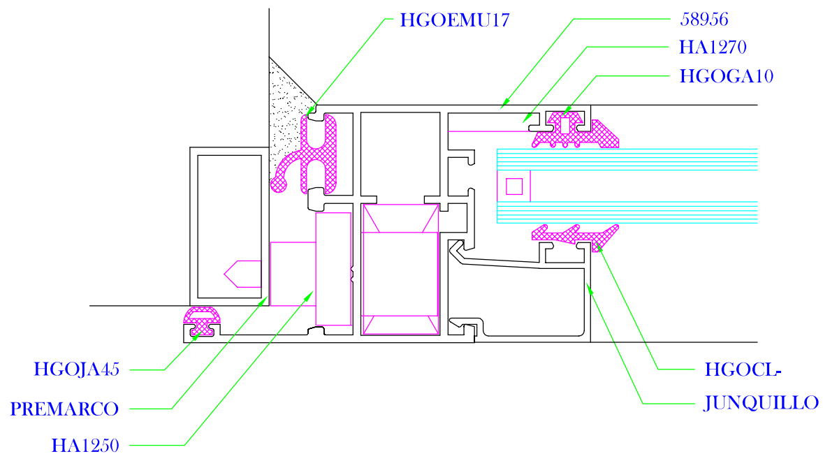
SECCIÓN LATERAL MARCO FIJO
