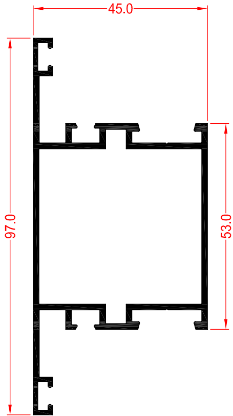
62285 TRAVESAÑO DE CERCO (97)
