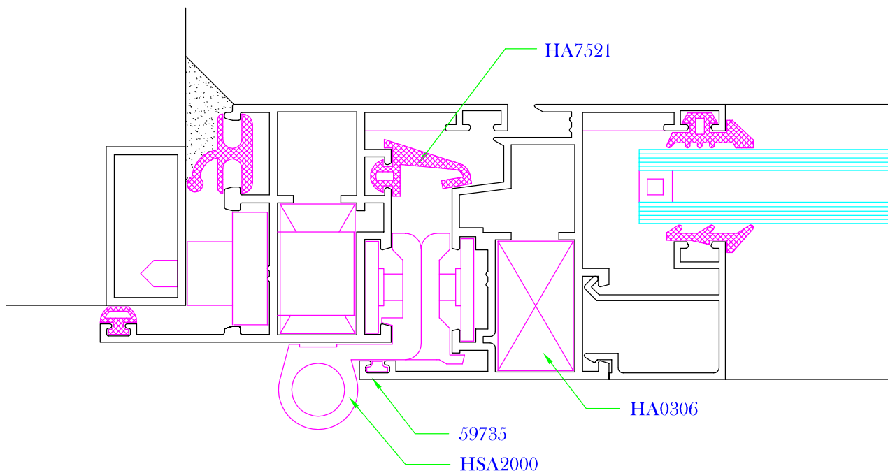
SECCIÓN LATERAL VENTANA
