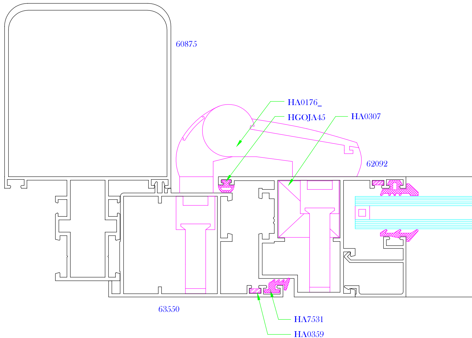
INVERSOR CON BISAGRA EXTERIOR
