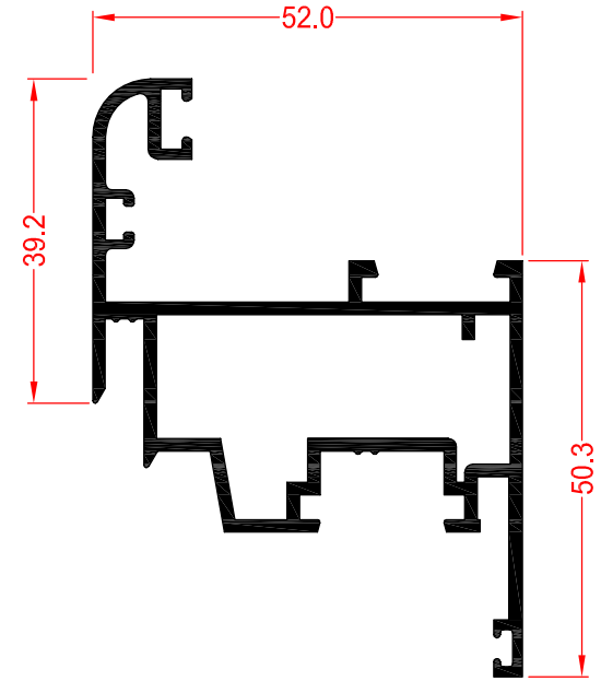
70532 HOJA CURVA VENTANA (15)
