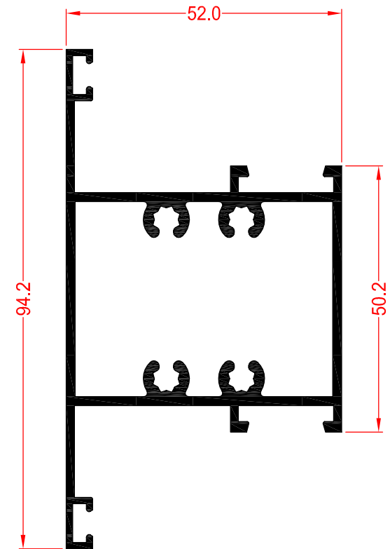
61142 TRAVESAÑO DE HOJA (94)
