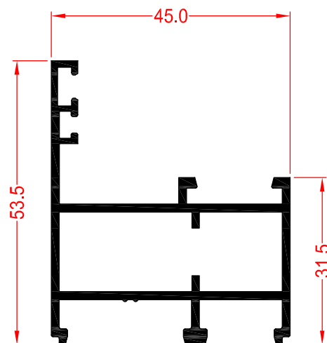
62091 CERCO VENTANA APERT. EXT.
