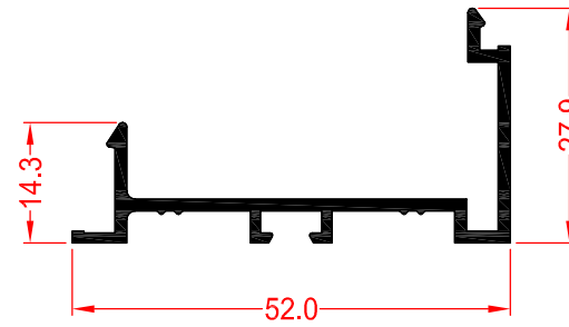
58962 CIERRE INFERIOR
