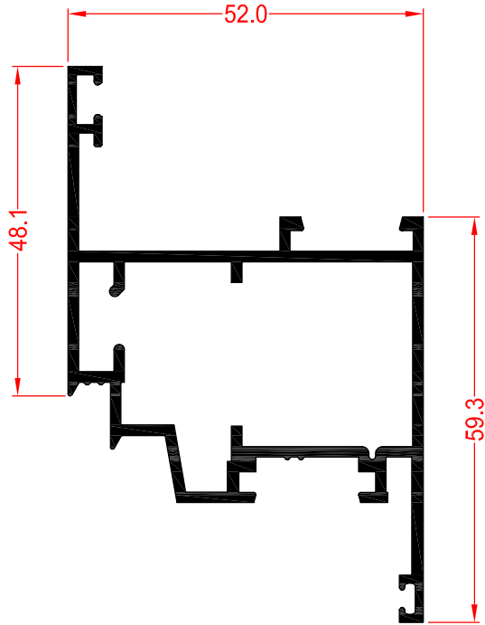
59736 HOJA PUERTA (27)
