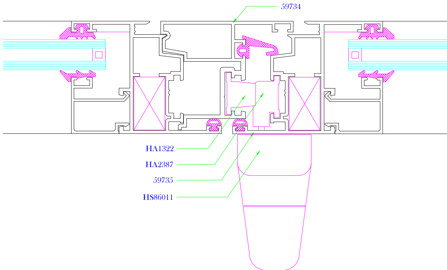
SECCIÓN CENTRAL VENTANA DE 2 HOJAS
