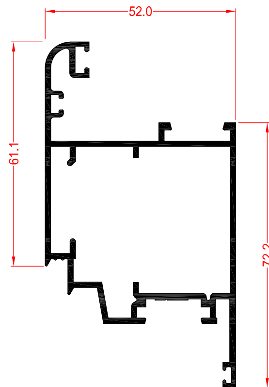
65188 HOJA PUERTA CURVA (40)
