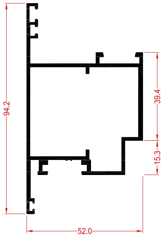
61189 HOJA PUERTA APERT. EXT.
