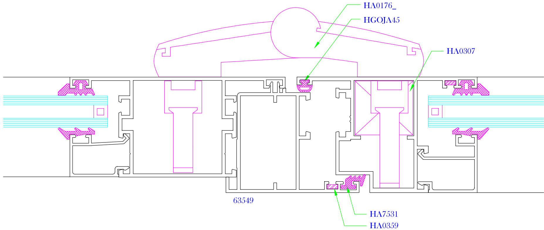
INVERSOR CON BISAGRA EXTERIOR
