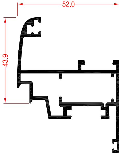
70364 HOJA CURVA VENTANA (15)
