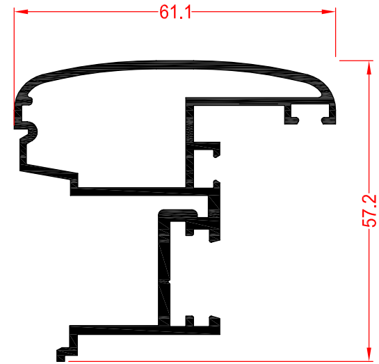
70365 INVERSOR CURVO
