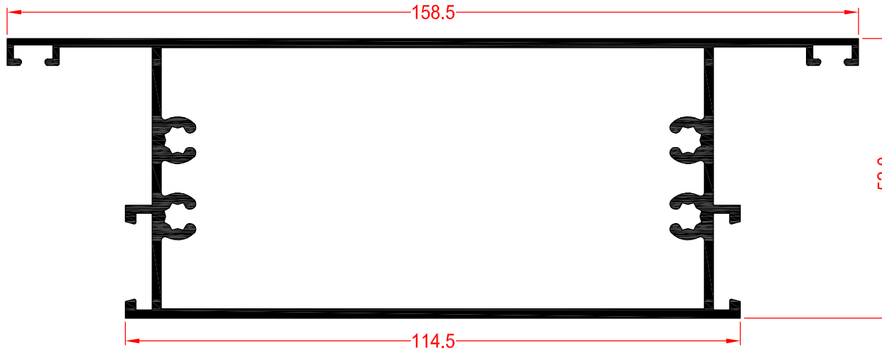
58953 TRAVESAÑO DE HOJA (158.5)
