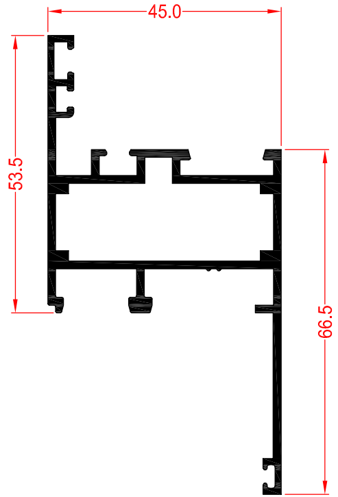
70530 CERCO VENTANA CON SOLAPE
