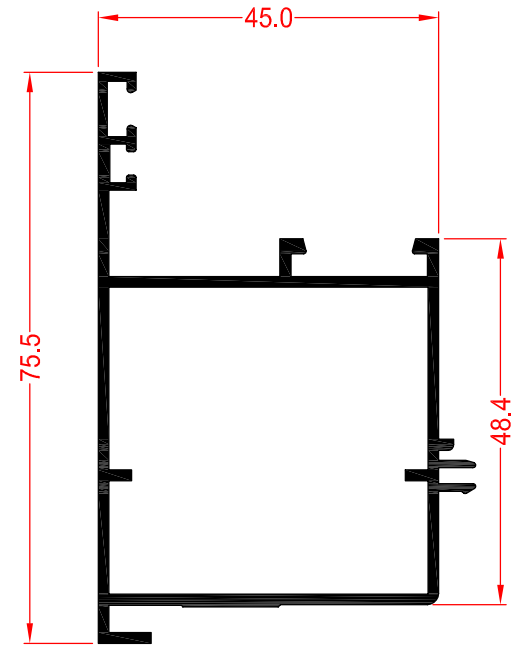
63550 INVERSOR CAMBIO APERT. EXTERIOR
