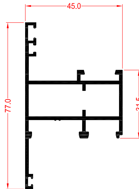
61141 CERCO VENTANA APERT. EXT. SOLAPE
