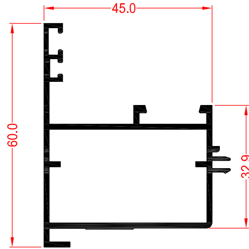
63549 INVERSOR CAMBIO APERT. EXTERIOR
