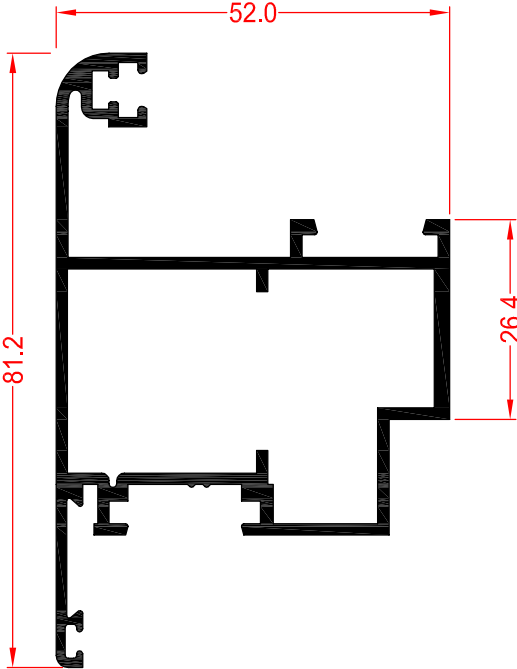
67527 HOJA CURVA APERT. EXT.
