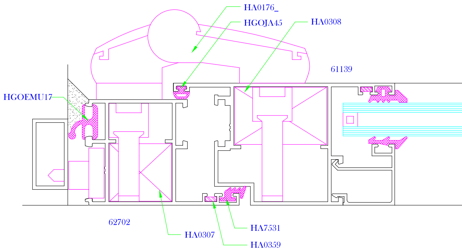
NUDO ESTÀNDAR BISAGRA EXTERIOR
