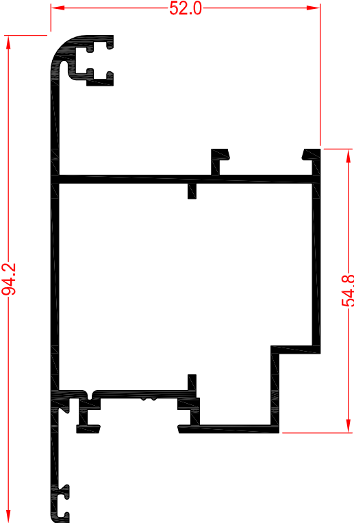
70215 HOJA CURVA APERT. EXT.
