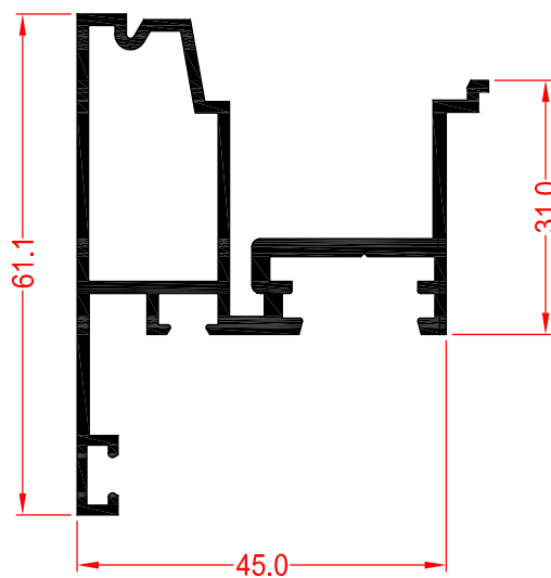
59734 INVERSOR
