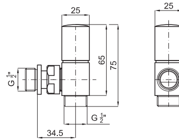
Válvula quadrada 1/2" + racord para tubo decobre Ø15
