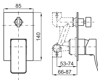
ARQUITECT Parte externa monocomando encastre baño/duche
