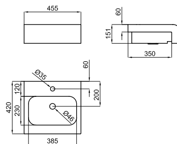
Lavatório 46x42 cm. semi-engaste com trasbordamento de água.
