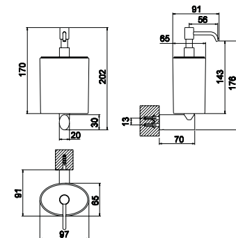
Doseador para a pared
