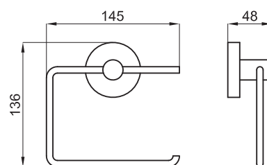
Portarolo sem tampa
