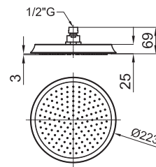
DINASTY - Pinha chuveiro 22 cm., com rótula (1) (2).
