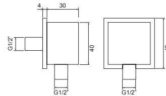
SQUARE - Toma de água de parede para tubo flexível
