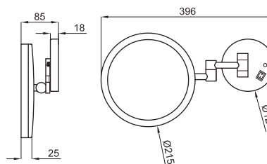
Espelho aumento 2 braços a parede com luz LED
