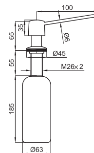
Doseador de sabao encastre bancada
