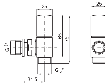
Detentor quadrado 1/2" + racord 1
