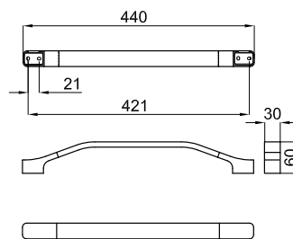
Toalheiro barra 44 cm.
