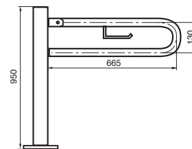
Barra duplo rebatível vertical com pé e portarolo
