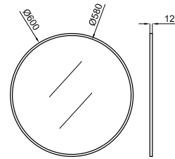
Espelho Ø60 cm. com moldura lacada
