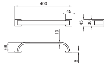
Toalheiro barra 40 cm.
