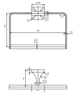
Toalheiro argola lavatório
