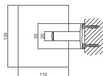
Portarolo com tampa
