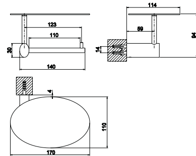
Portarolo com tampa
