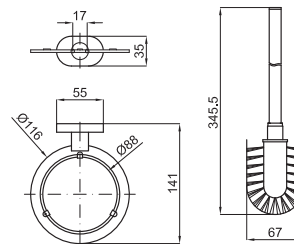
Portapiçaba para a parede
