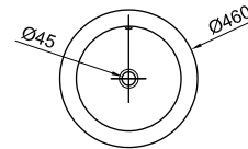
XL BOLD - Lavatório Ø46 cm. apoio com trasbordamento de agua
