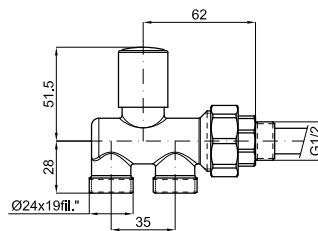
Válvula monotubo vertical (3)
