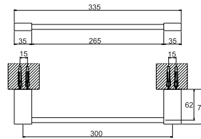
Toalheiro barra 30 cm.
