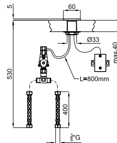
Kit sensor remoto com embelezador quadrado
