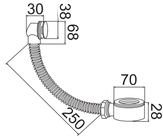
Jogo transbordamento de agua
