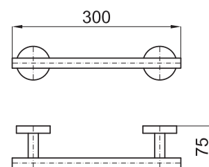
Pega banheira 30 cm.
