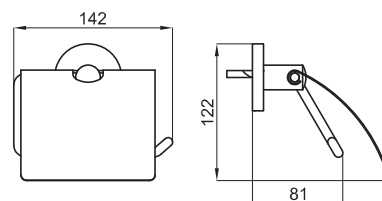
Portarolo com tampa
