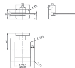
Saboneteira para a parede
