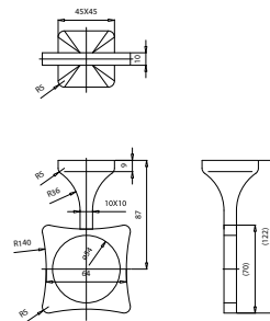
Saboneteira para a parede
