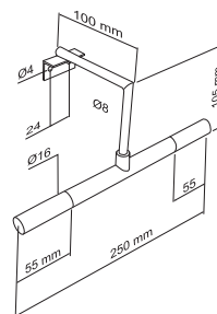
LLUM - Applique 2x20W G4 12V + transformador. Montagem sobre espelho canto polido, moldura aluminio e espelho táctil
