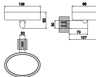
Saboneteira para a parede
