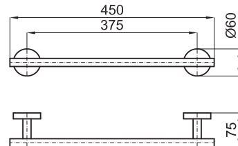
Toalheiro barra 45 cm.
