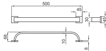
Toalheiro barra 50 cm.
