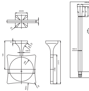
Portapiçaba para a parede
