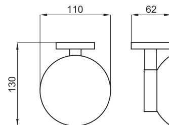
Saboneteira a parede
