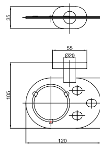
Porta-objetos para a parede
