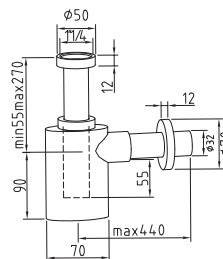
LIBRA - Sifão garrafa lavatório
