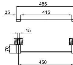
Toalheiro barra 45 cm.
