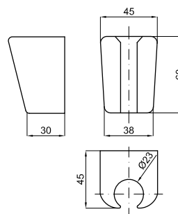
Suporte fixo chuveiro de mão
