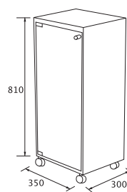
Armário ao chão rodas 1 porta 35x30x81h cm.
