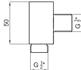
LIBERTY - Toma de água de parede para tubo flexível
