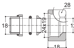
Racord nivelite 24x19x12 cm.
