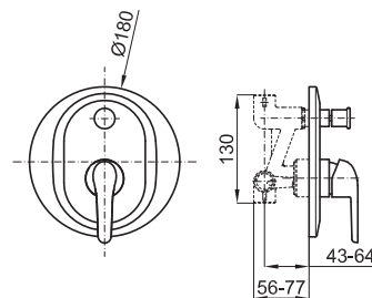
MINI PLUS Parte externa monocomando encastre baño/ducha
