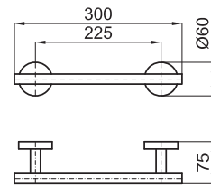
Toalheiro barra 30 cm.
