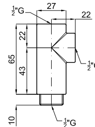
Racord "T" para radiador misto (2)
