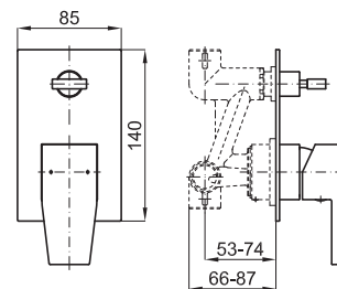
ACRO N Parte externa monocomando encastre baño/duche
