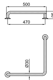
Assa parede 50x50 cm. 90°
