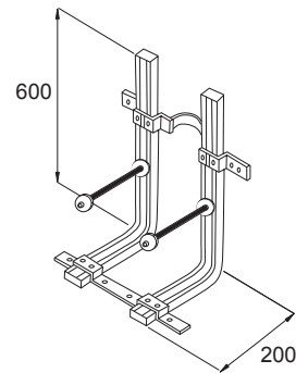
Suporte sanita - bidé suspenso para instalar engastado em parede sólida.
