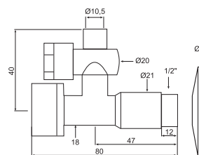
AERO - Torneira de passagem com filtro desmontável
