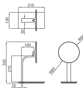
Espelho aumento orientável apoio
