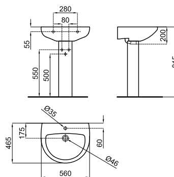
Lavatório 56 cm. com trasbordamento de água e fixações 100041225 - N421040000.
