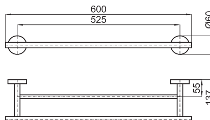
Toalheiro barra duplo 60 cm.
