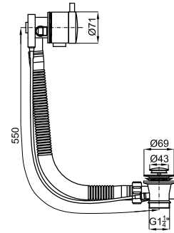
Trasbordamento dem agua com torneira de bañeira
