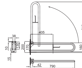
Barra rebatível vertical 80 cm. com portarolo
