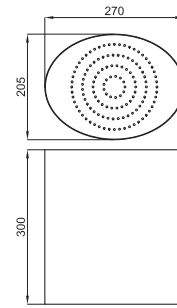
Pinha chuvaireiro instalação no tecto 30 cm.
