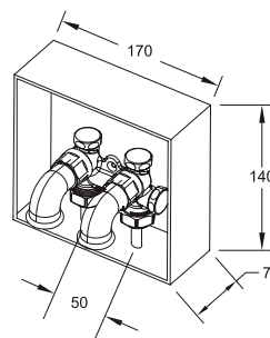
TETRIS - Válvula engaste à parede
