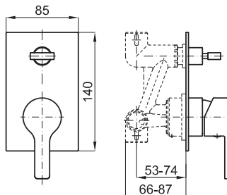
URBAN Parte externa monocomando encastre baño/duche
