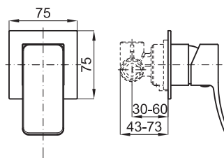
ARQUITECT Parte externa monocomando encastre duche
