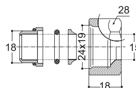
Racord nivelite 24x19x15 cm.
