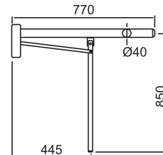
Barra rebatível vertical parede ligeira
