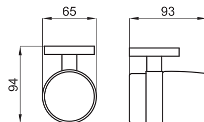
Porta-objetos a parede
