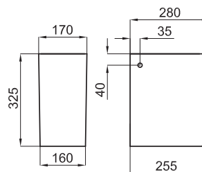
Meia coluna para lavatório 60 cm. (100080133 - N380000004) e pia 50 cm. (100097414 - N380000017) com fixações 100041212 - N420150000
