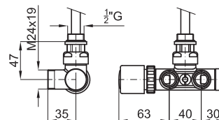
Válvula monotubo horizontal (3)
