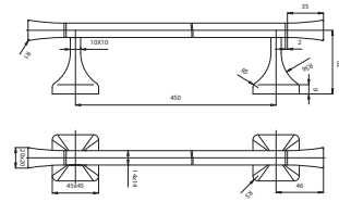
Toalheiro barra 45 cm.
