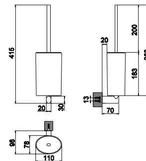
Portapiçaba para a parede
