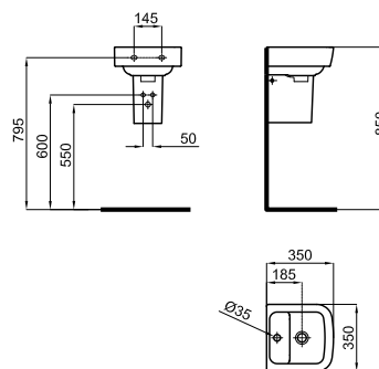
Lavamão suspensa 35 cm. com transbordamento de água e fixações 100041225 - N421040000.
