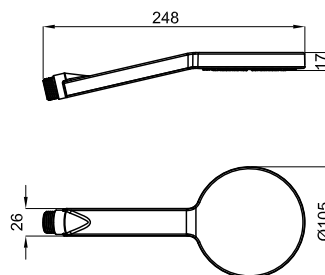
HOTELS - Chuveiro de mão 1 posição com sistema AIR ECO
