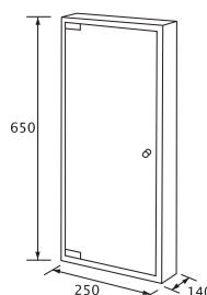
Armário suspenso 1 porta 25x14x65h cm.
