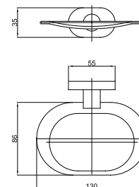
Saboneteira para a parede
