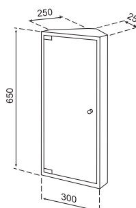
Armário suspenso ângulo 1 porta espelho 25x25x65h cm.
