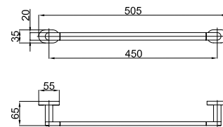
Toalheiro barra 45 cm.
