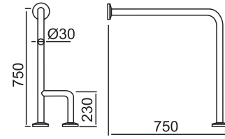
Barra parede / chão e apoios
