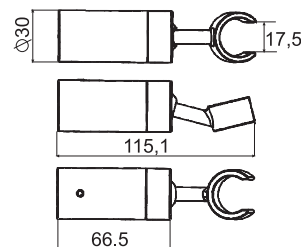
MINIMAL - Suporte orientável chuveiro de mão
