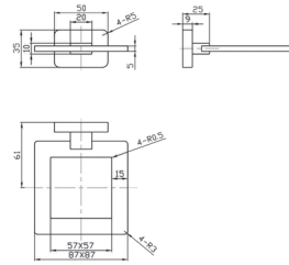
Porta-objetos para a parede
