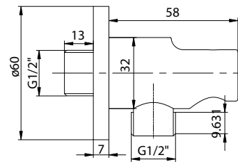
MINIMAL - Suporte chuveiro de mão a parede com toma de água.
