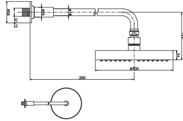
FUTURE - Kit pinha chuveiro 20 cm.+brazo
