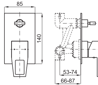
ACRO N OPEN Parte externa monocomando encastre baño/ducha
