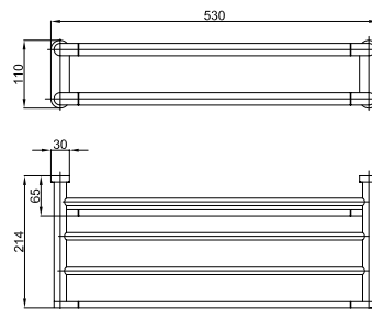
Toalheiro de prateleira
