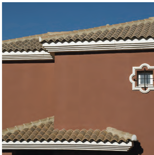
duna flameada teja cerámica mixta de: 472 x 282 mm. / coloración en masa: salmón / peso: 3625 gr. / 1,3 piezas por m 2
