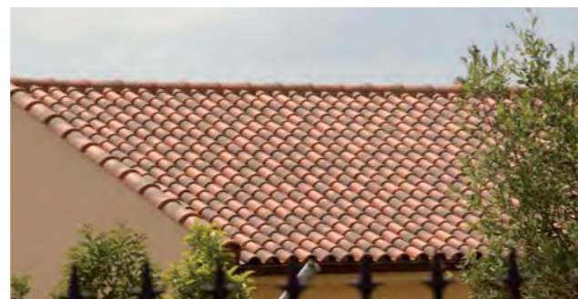
roja envejecida teja cerámica occitania de: 466 x 273 mm. / coloración en masa: rojo / peso: 3840 gr. / 12,2 piezas por m 2
